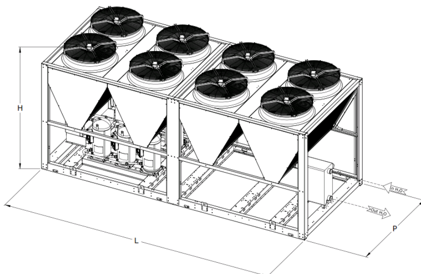
Figura 2.6: Disegno dimensionale generico serie RAE N MC Kc
